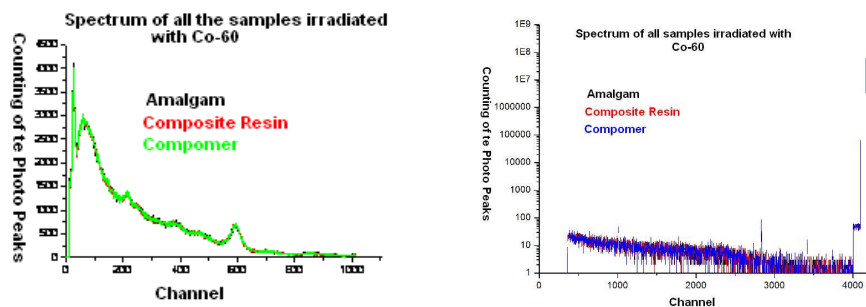
Figura 4: Espectros de todas as amostras analisadas em 2001 e 2009, respectivamente.
