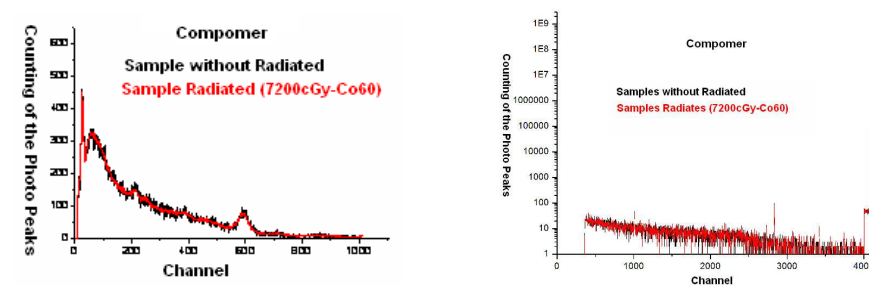
Figura 3: Espectrometria gamma das amostras de compômero obtidas em 2001 e 2009, respectivamente.
