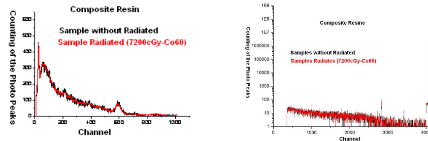
Figura 2: Espectrometria gamma das amostras de resina composta obtidas em 2001 e 2009, respectivamente.
